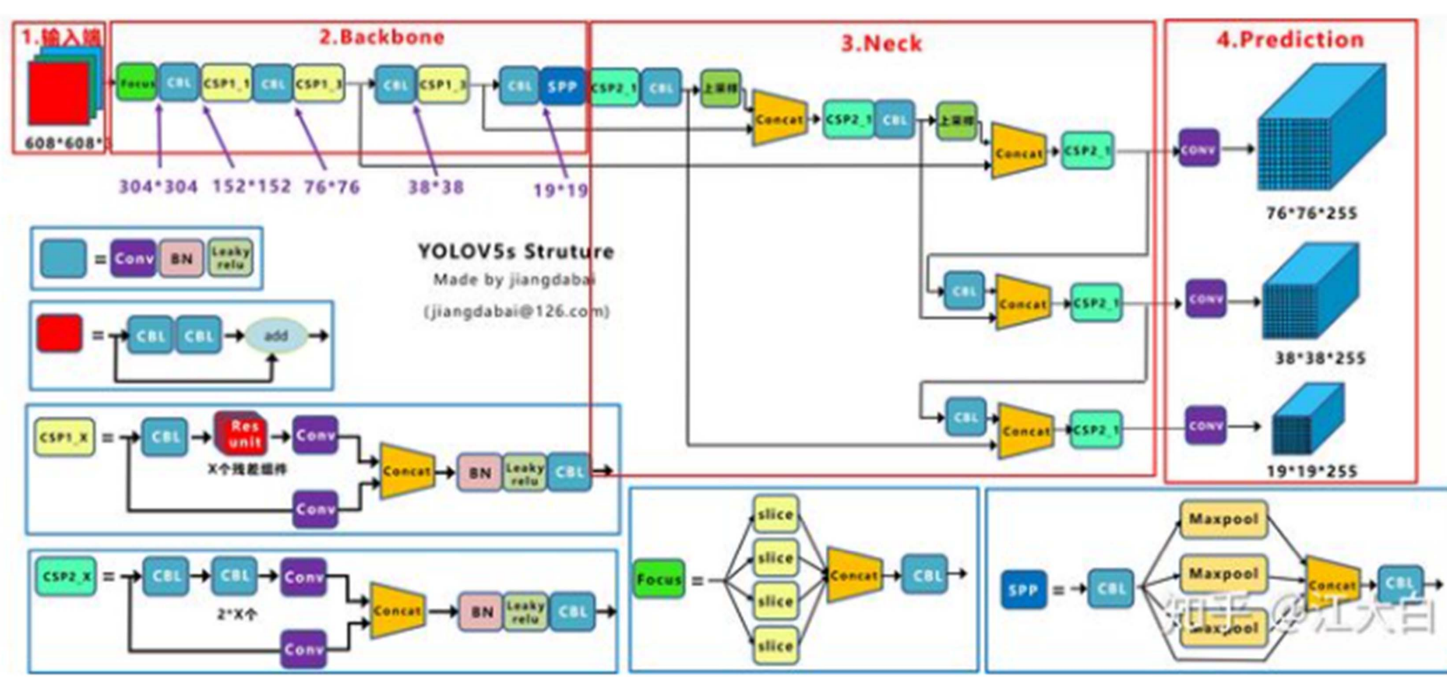
YOLOV5 架構
